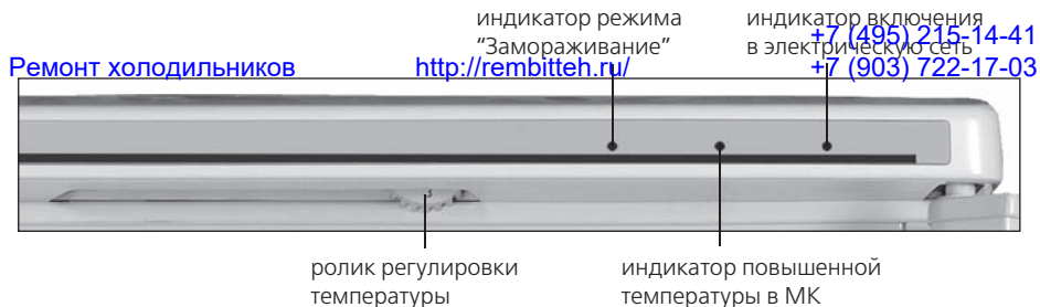
Рисунок 6 — Световая индикация холодильника однокомпрессорного (со звуковой сигнализацией)
